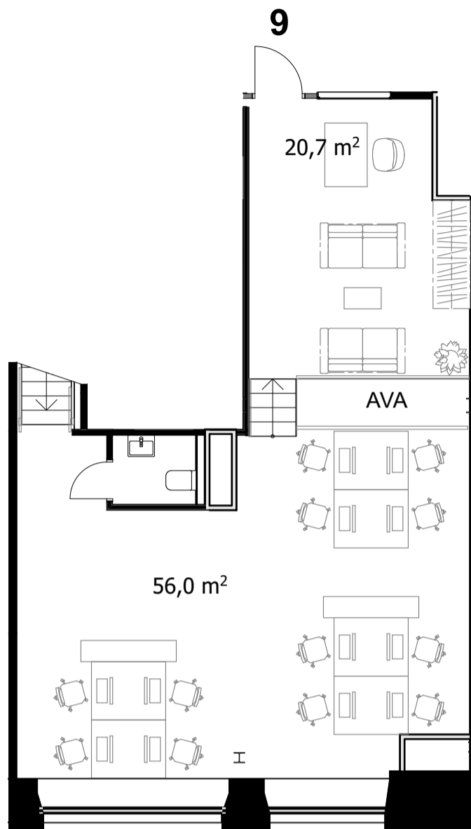
2. KORRUS
